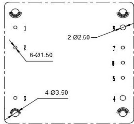
推荐PCB开槽尺寸
