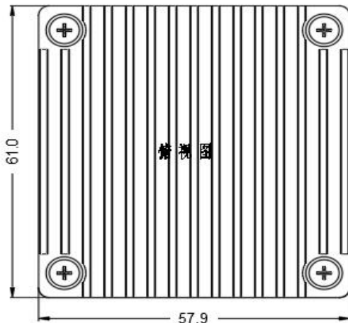
标准型+散热器
